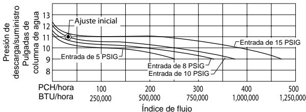
Regulador de segunda etapa serie LV4403B
